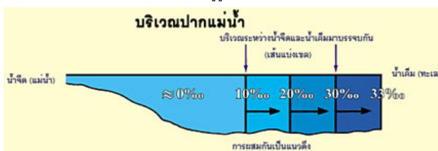
รูปที่ 14: ส่วนที่เป็นเส้นตั้งตรง แสดงให้เห็นถึงความเค็ม (ส่วน ต่อกว่า) หนึ่งใน พันเปอร์เซ็นต์) ในบริเวณปากแม่น้ำ เราจะเห็นการแบ่งเขต (เขตการแบ่งแยก) ที่กั้นระหว่างน้ำจืดกับน้ำเค็ม (Introductory Oceanography ของ Thurman หน้า 301 ฉบับปรับปรุงเพิ่มเติมเล็กน้อย)
