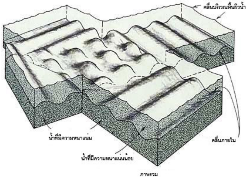
รูปท 16: คลื่นใต้น้ำบริเวณที่มีชั้นน้ำสองชั้นซึ่งมีความหนาแน่นต่างกันมาประสานกัน สายหนึ่งจะมีความหนาแน่นมากกว่า (สายที่อยู่ต่ำกว่า) ส่วนอีกสายหนึ่งจะมีความหนาแน่นที่น้อยกว่า (สายที่อยู่ด้านบน) ( Oceanography ของ Gross หน้า 204)
