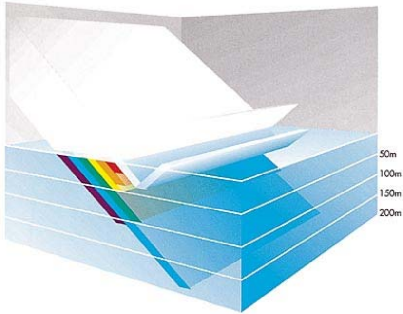
รูปที่ 15: ประมาณ 3 ถึง 30 เปอร์เซ็นต์ของแสงอาทิตย์จะสะท้อนบนผิวน้ำของท้องทะเล จากนั้น เกือบทั้งหมดของแสงที่เหลือจะถูกดูดซับหายไปทีละสีๆ ในระยะ 200 เมตรแรก ยกเว้นไว้แต่แสงสีน้ำเงิน ( Oceans ของ Elder และ Pernetta หน้า 27)
